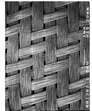
2/2 twill
